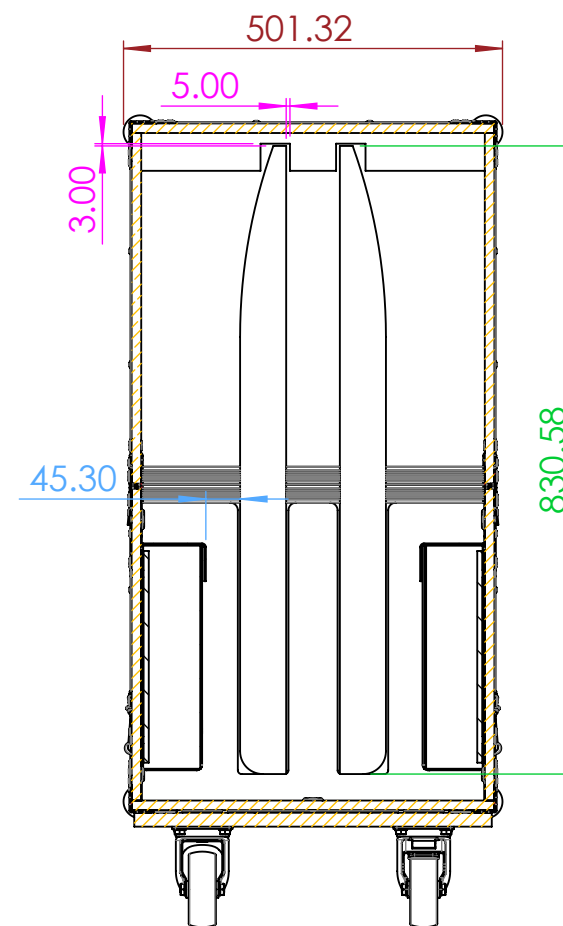
SECTION B-B SCALE 1 : 10
