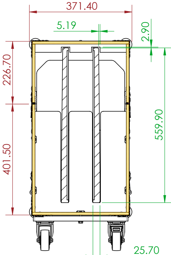
SECTION A-A
