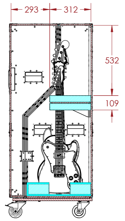
SECTION A-A SCALE 1 : 15
